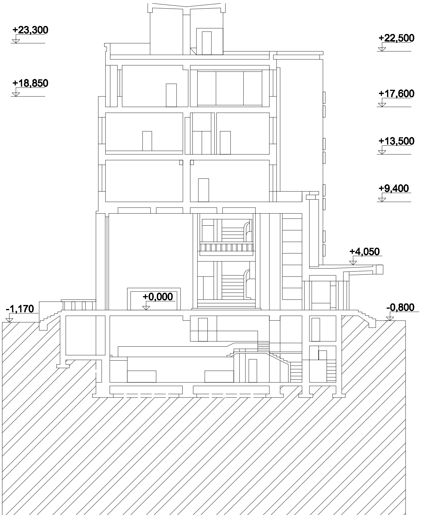
PRIECNY REZ M 1:200
