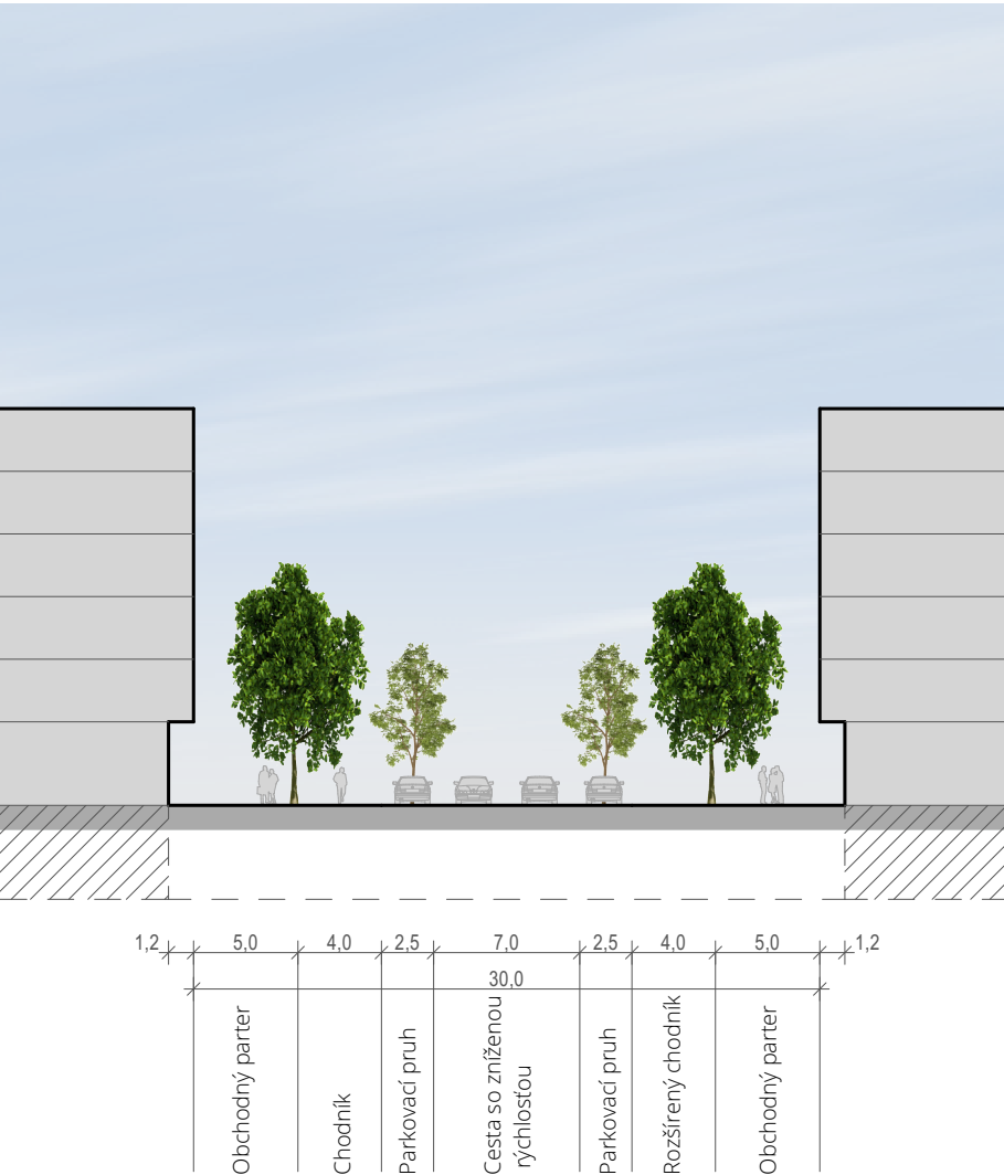
Uličné profil skludnenej ulice
