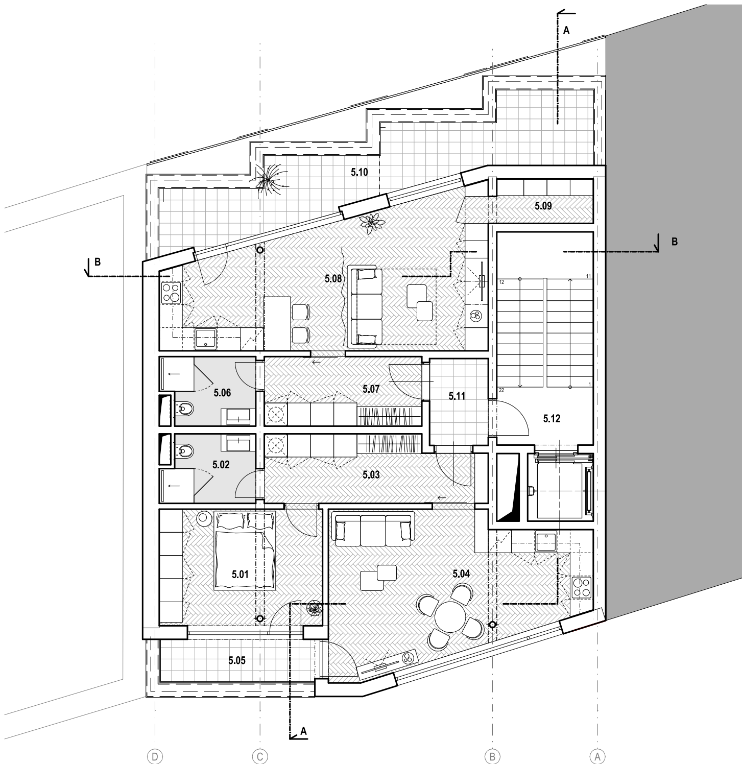
PÔDORYS 5. NADZEMNÉHO PODLAŽIA
