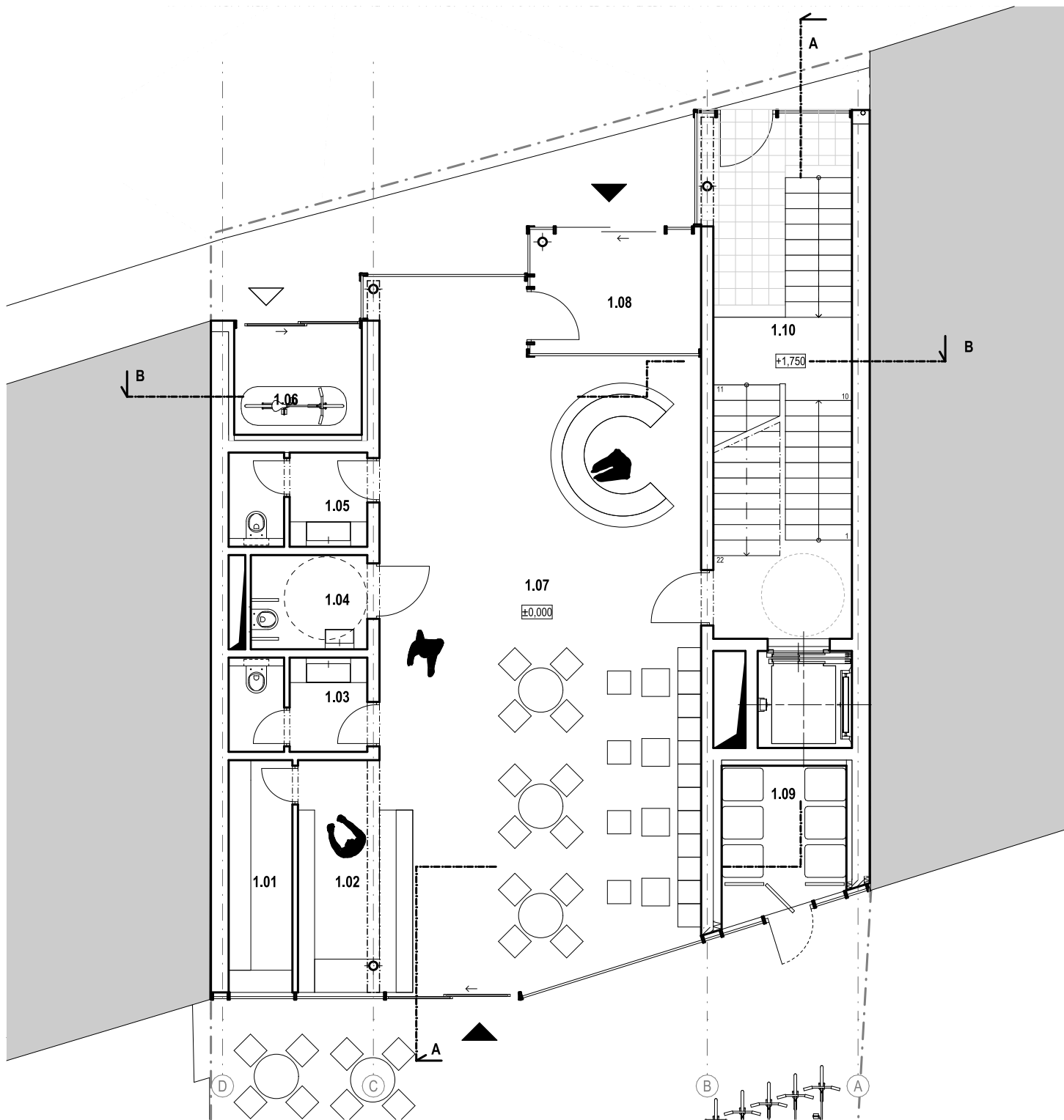
PÔDORYS 1. NADZEMNÉHO PODLAŽIA
