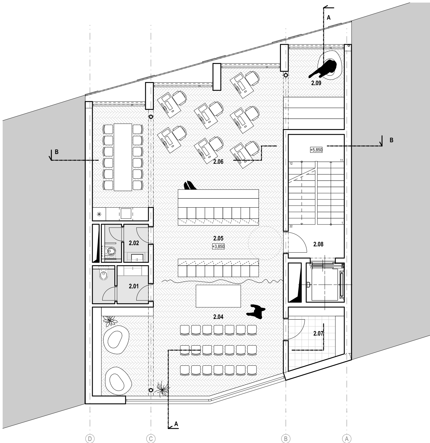
PÔDORYS 2. NADZEMNÉHO PODLAŽIA
