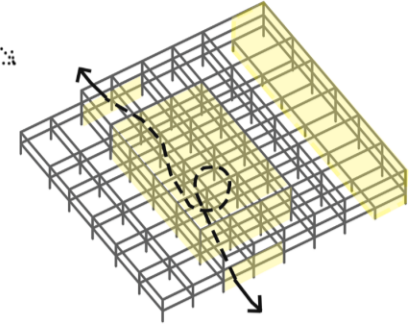
3. Odstránenie časti skeletovej konštrukcie.
