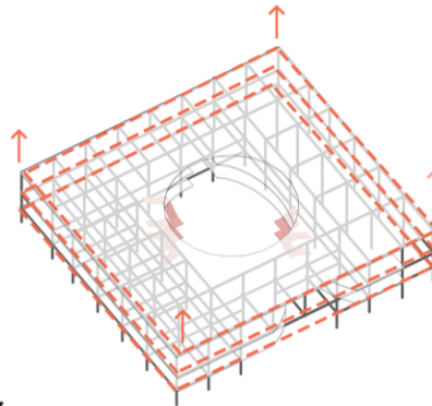
5. Zmena konštrukčných výšok.
