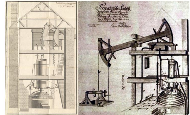
POTTEROV STROJ - NÁKRES
