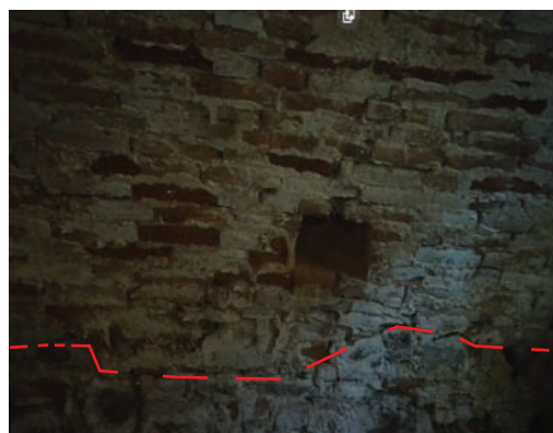
Napojenie plnej pálenej tehly na kamenné murivo
