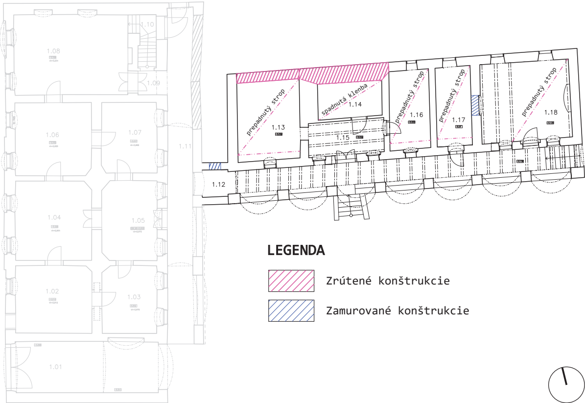
Prepadnutý trámový strop v dôsledku uhnitia záhlaví trámov (m.č. 1.13)
