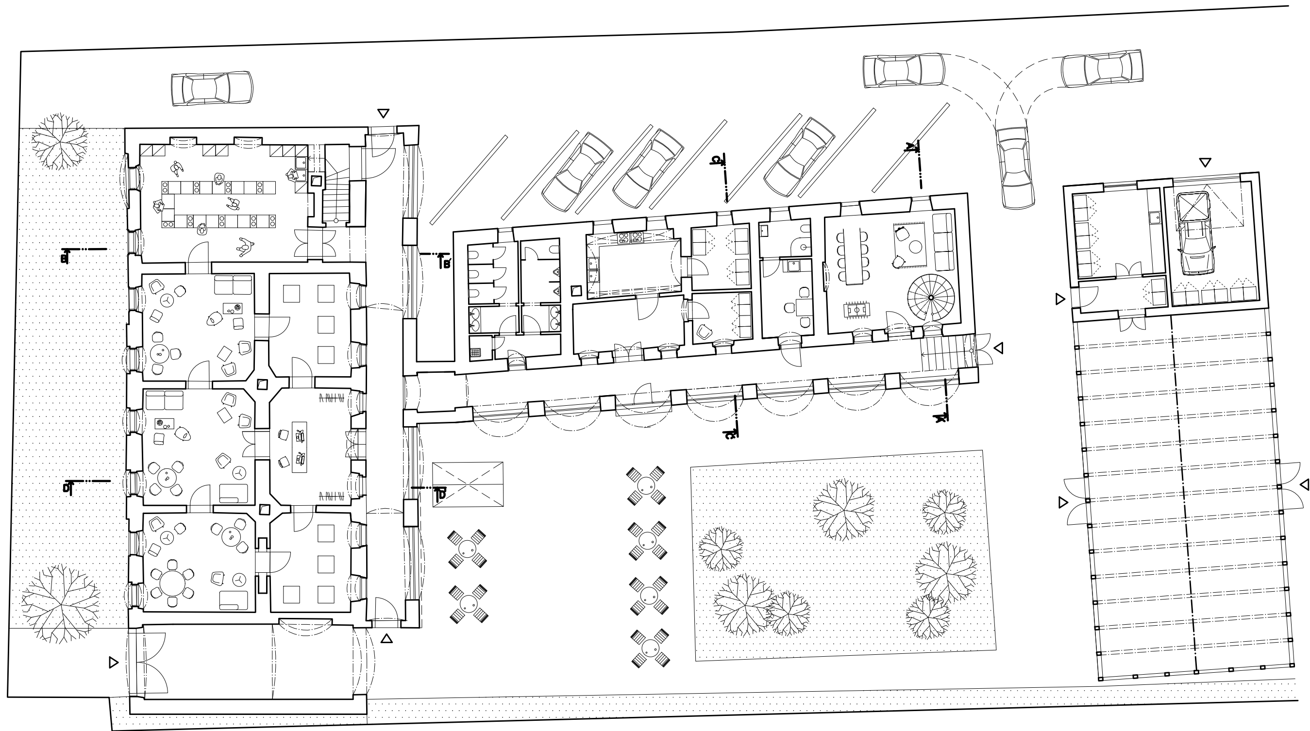
PÔDORYS 1NP
