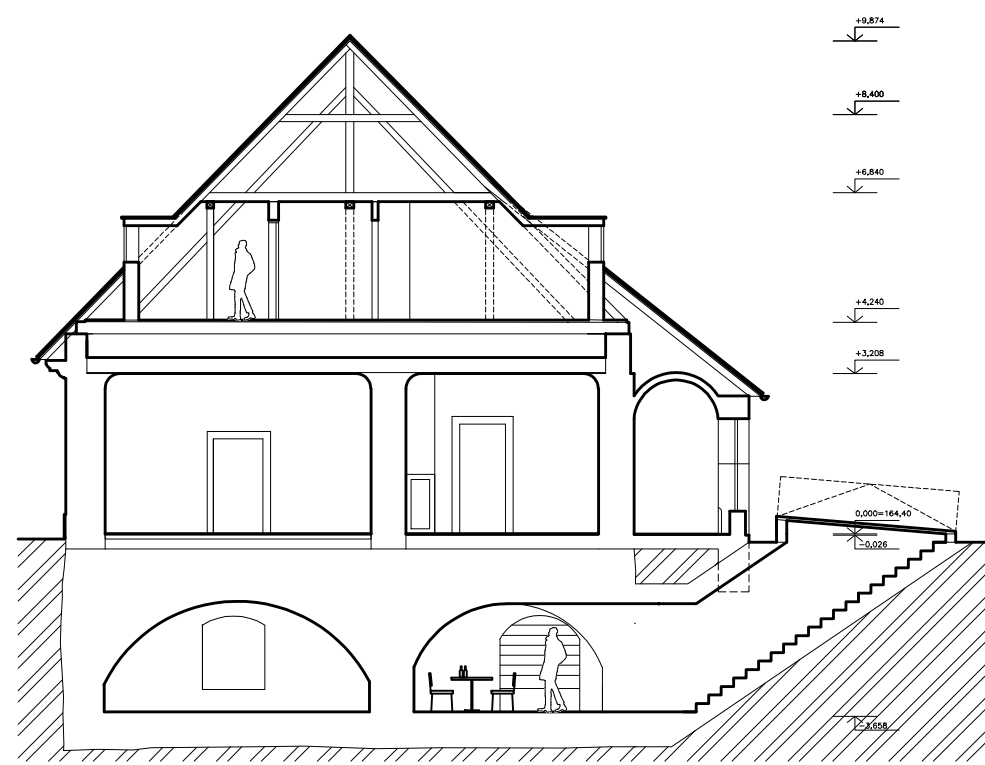
REZ DD M 1:100
