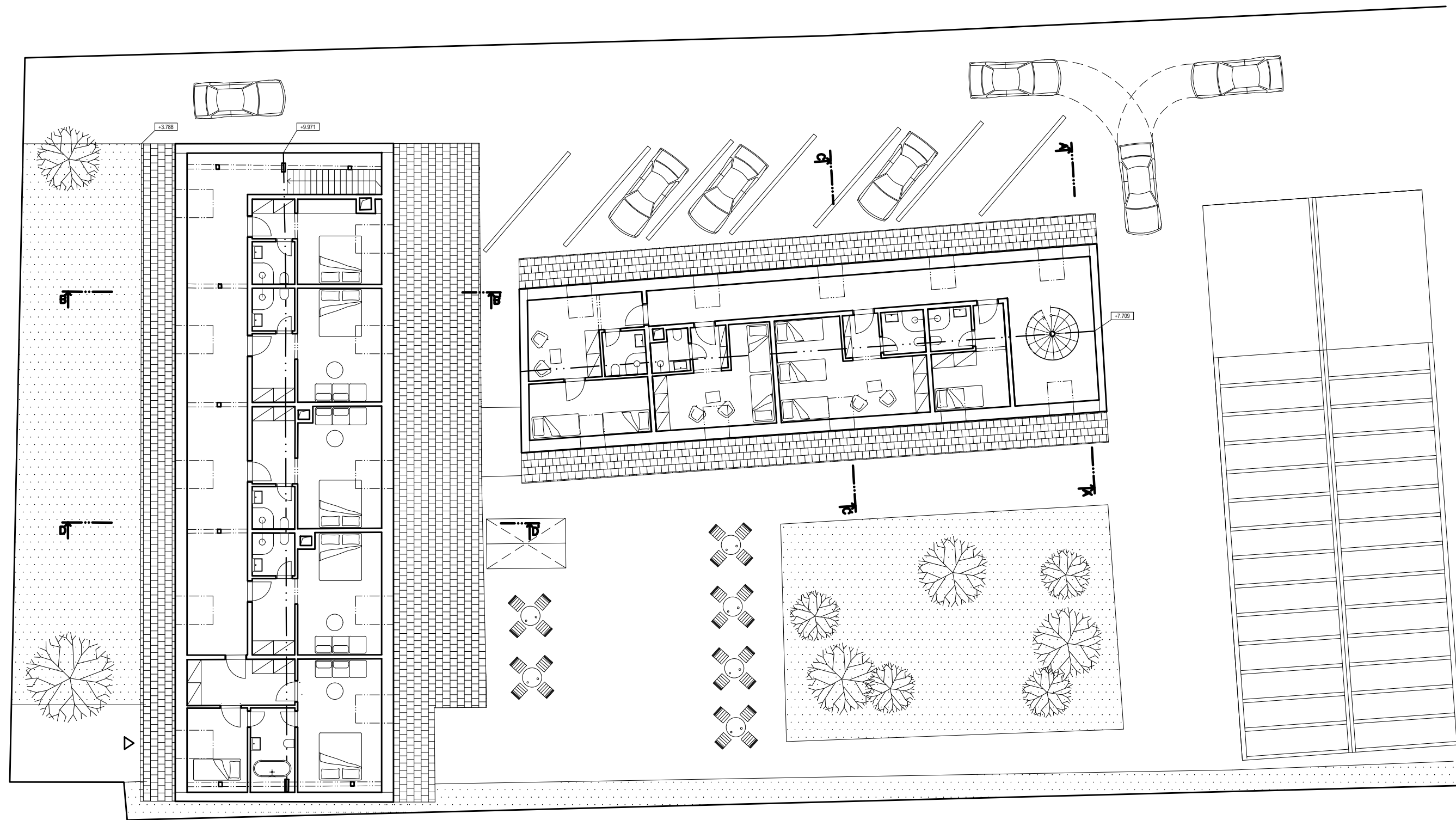
PÔDORYS KROVU
