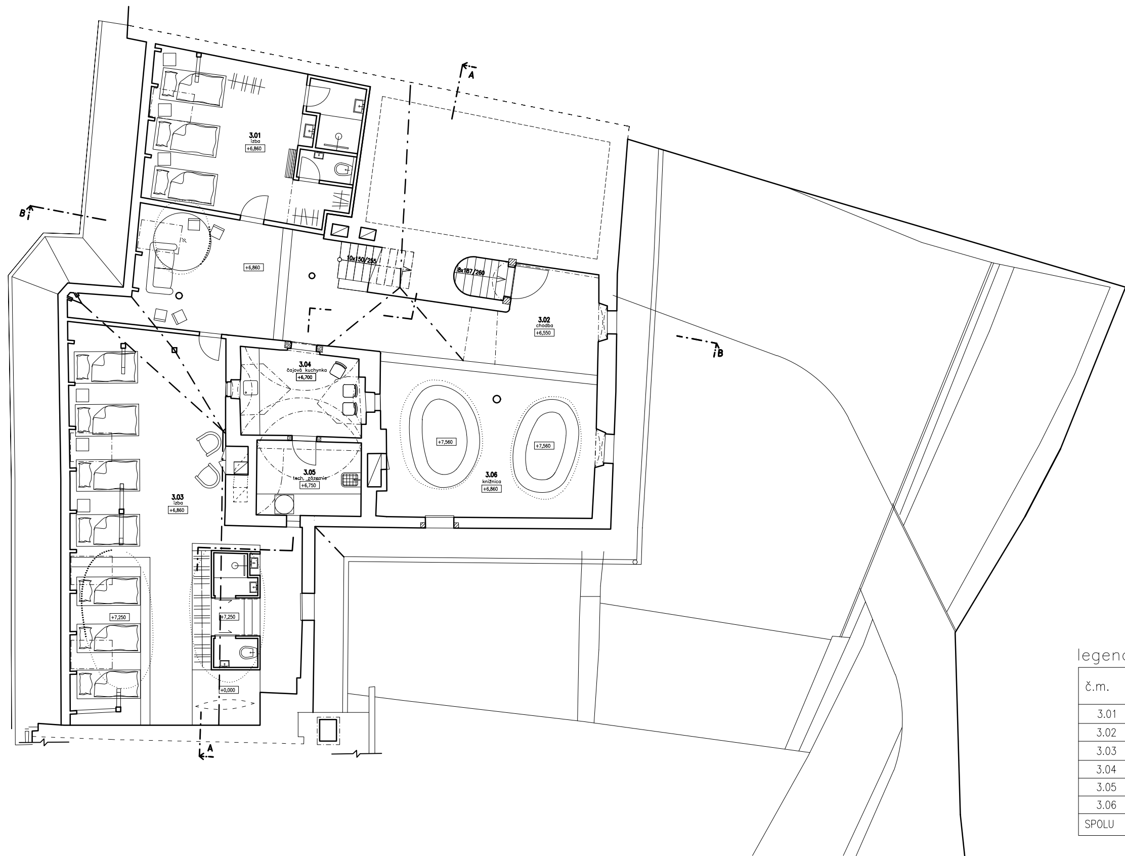
navrhovaný stav_3.nadzemné podlažie
