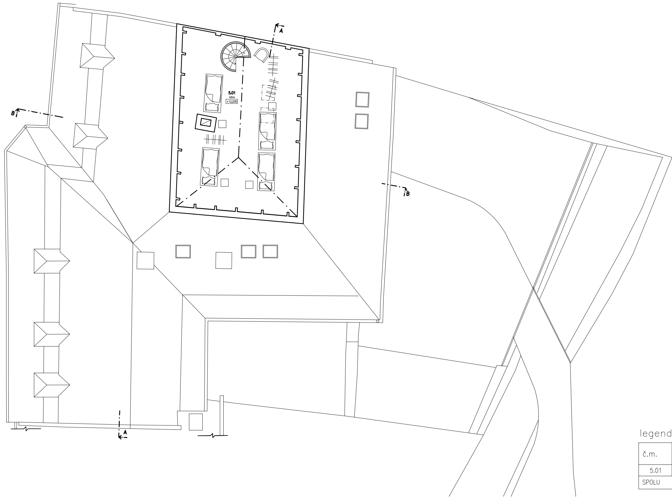
navrhovaný stav_5.nadzemné podlažie
