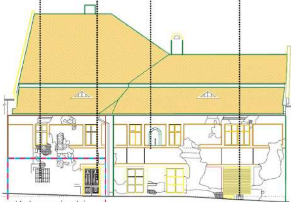
pohľad severozápadný
