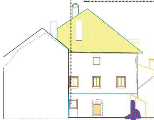
pohľad juhozápadný
