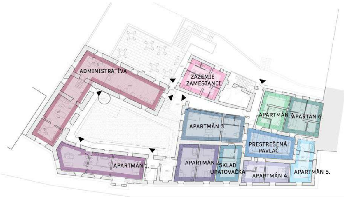
PÔDORYS 2.NP
