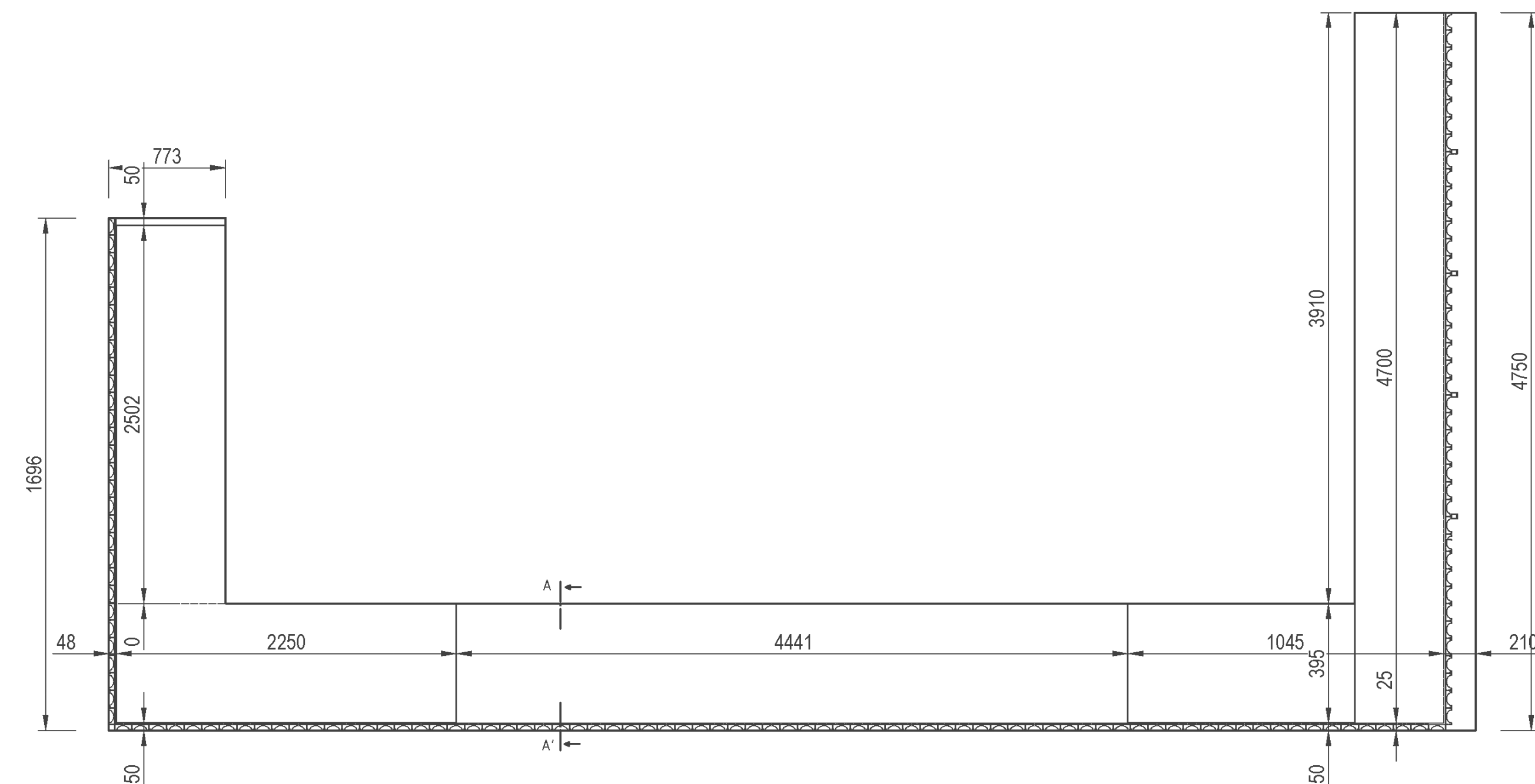
PÔDORYS
