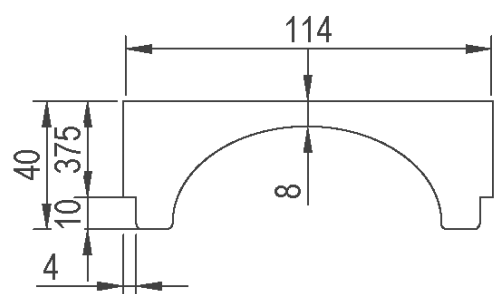
Profil obkladového panelu
