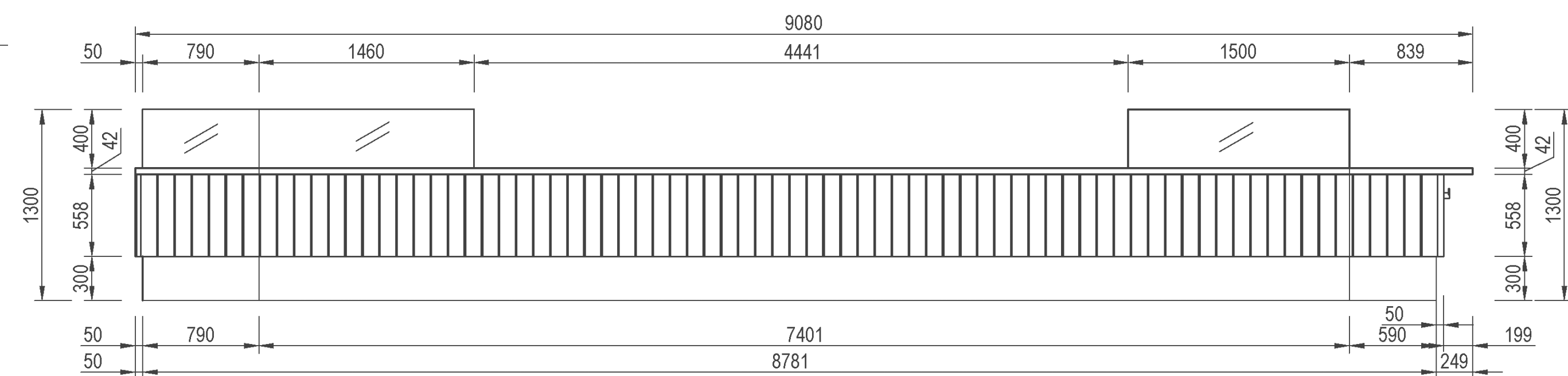
PÔDORYS
