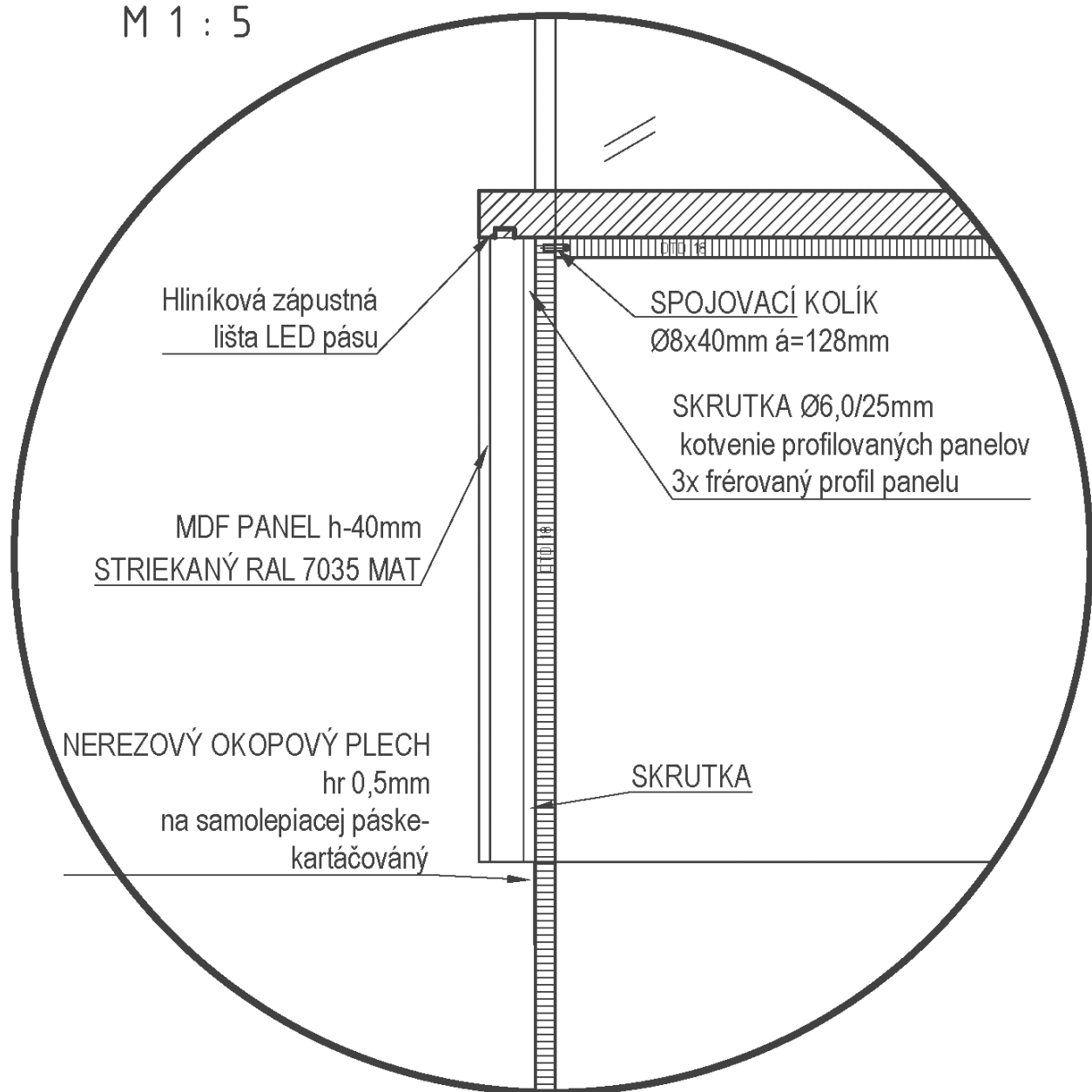
DETAIL A M 1 : 5
