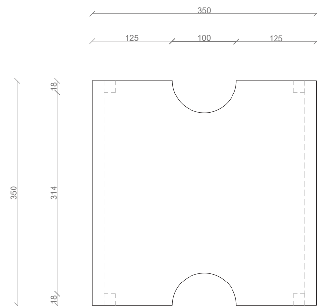
Nárys
