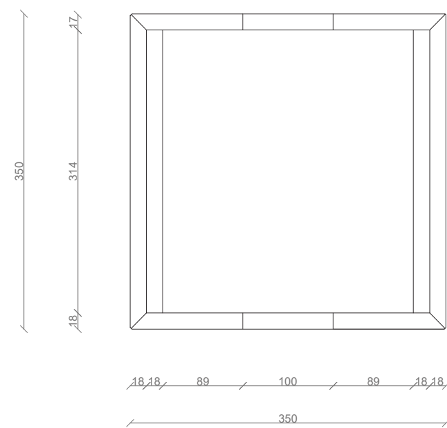
Pôdorys
