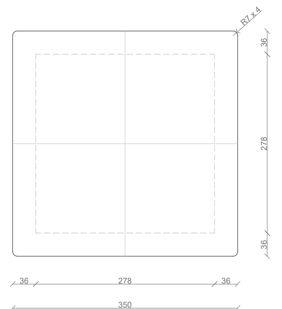
Pôdorys
