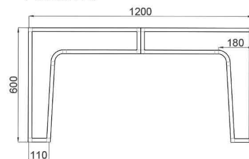
PÔDORYS
