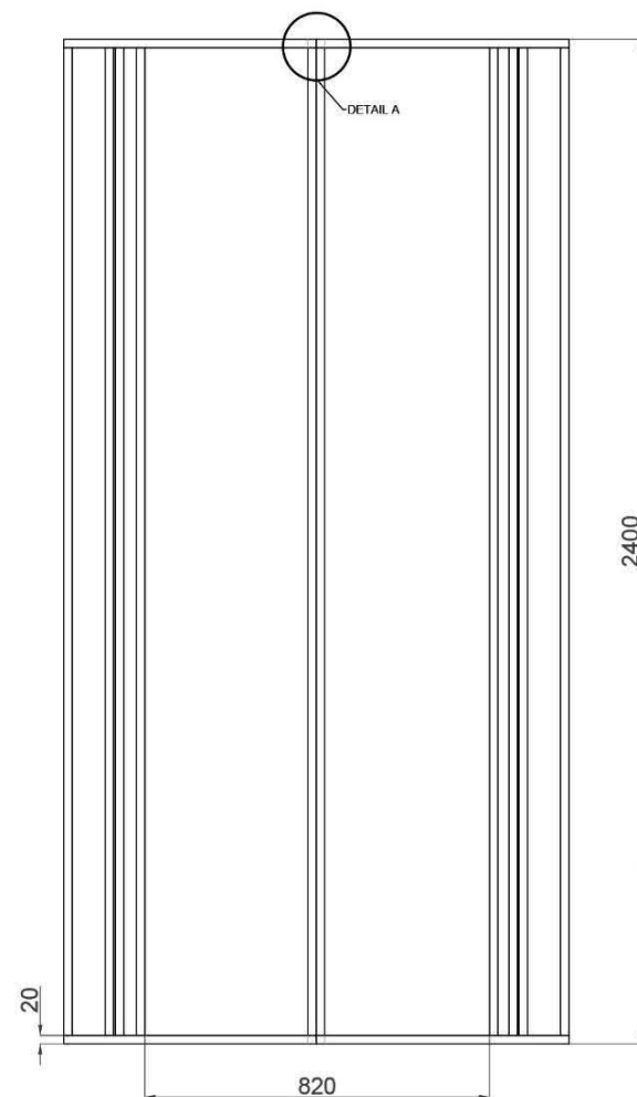
NÁRYS
