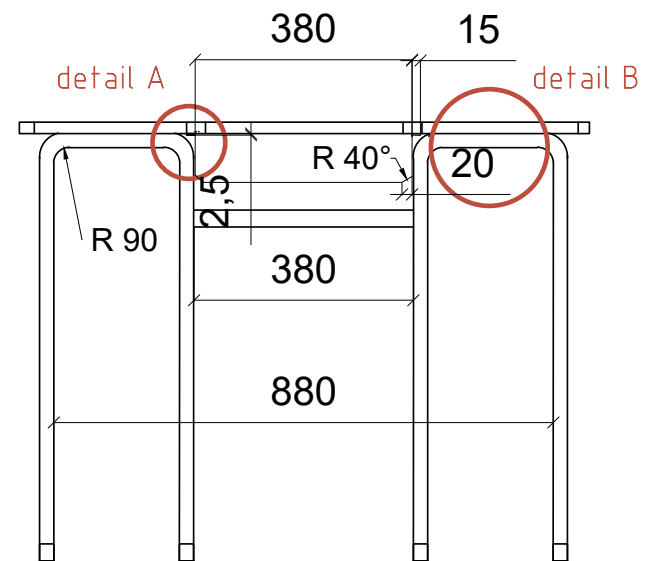
nárys
