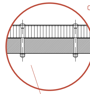
detail uchytenia oceľových tyčí o preglejkovú dosku
