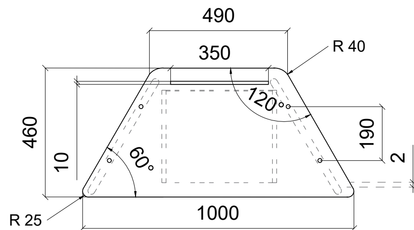
pôdorys
