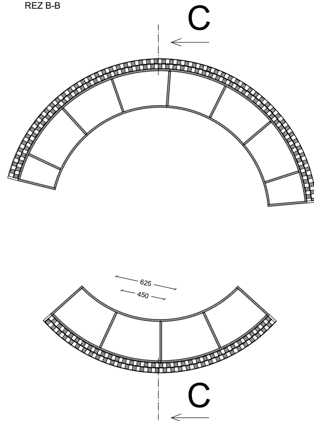
REZ B-B
