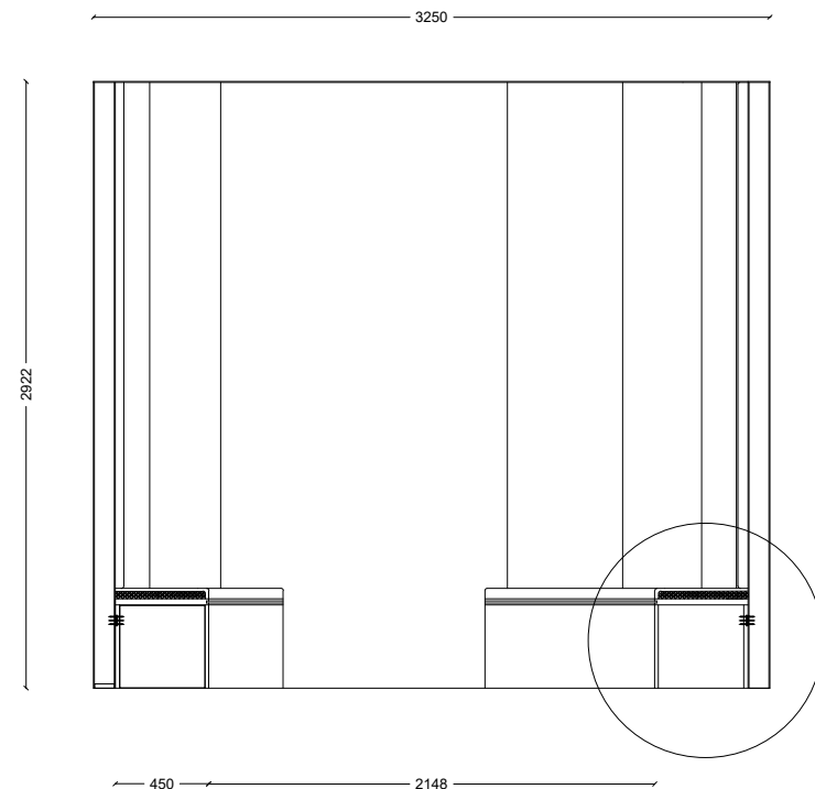
REZ C-C
