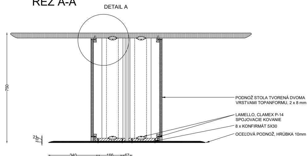
REZ A-A'
