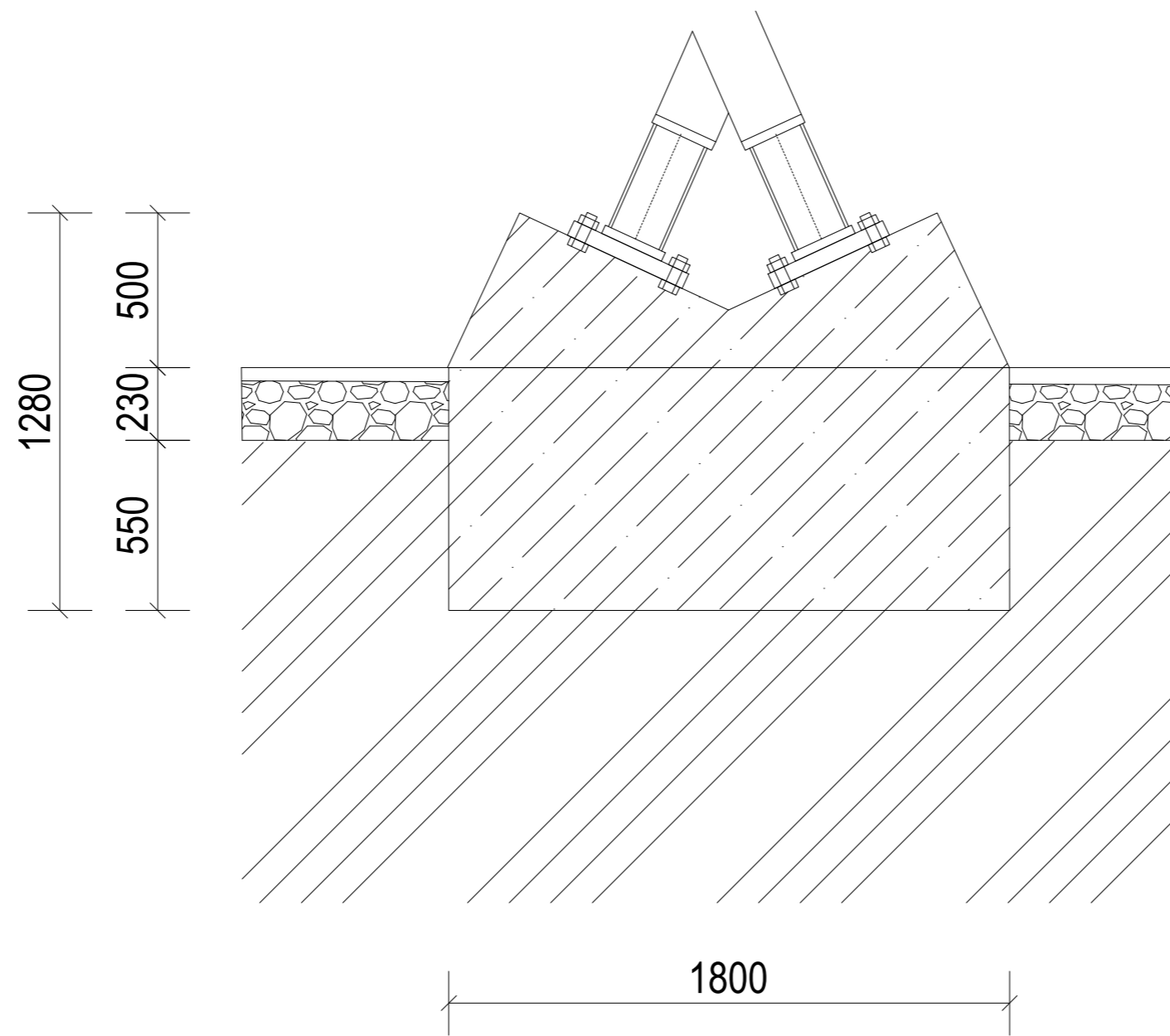
PLATŇA KP1 - 1KS 360 x 360 x 311 mm
