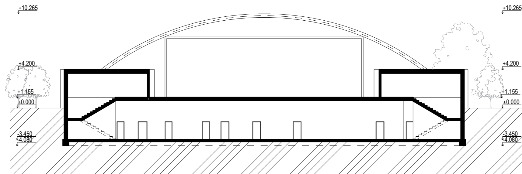
REZ D - D'
