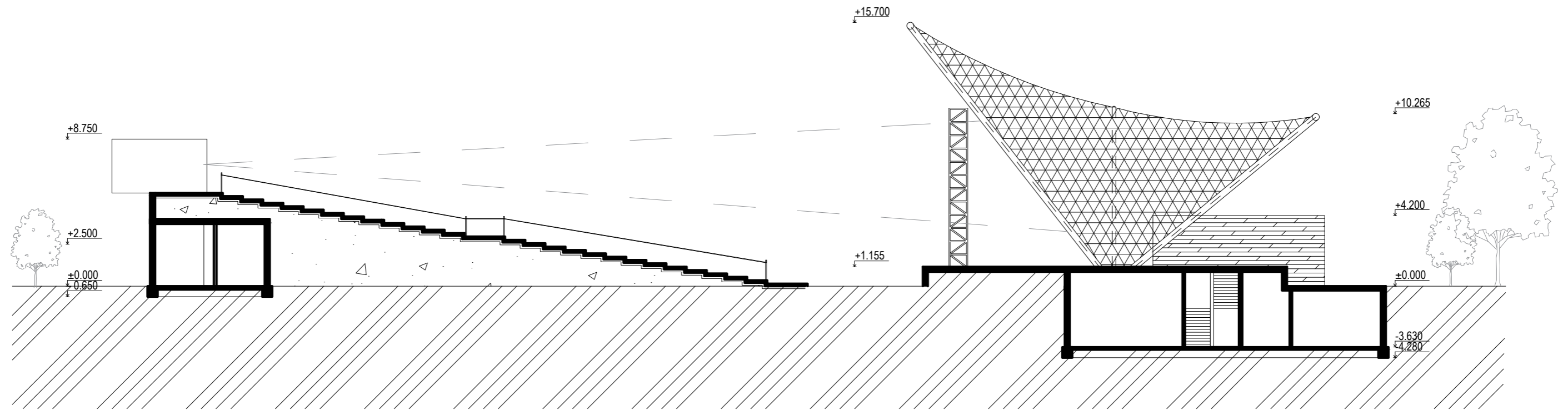
REZ A - A'
