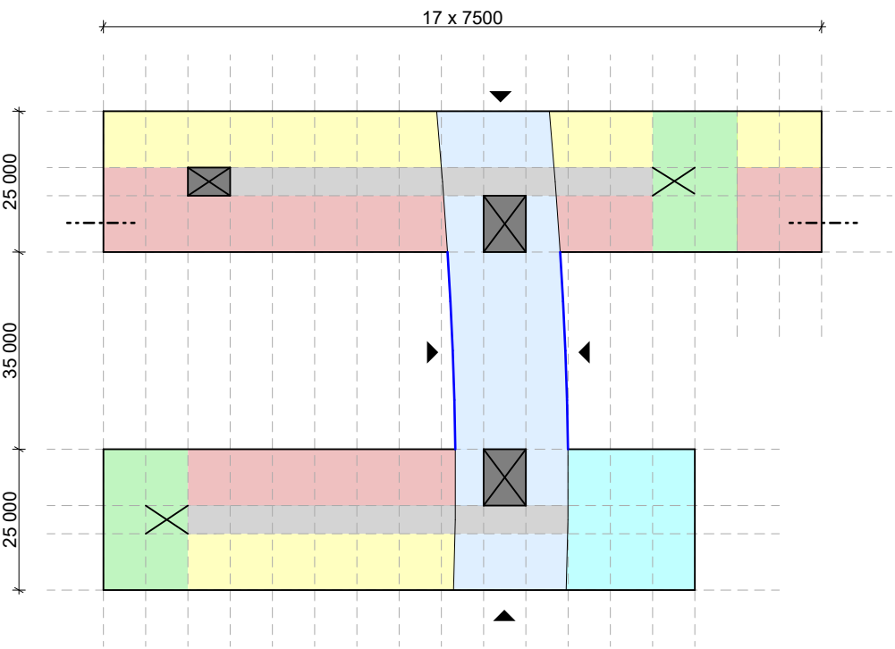
PÔDORYS 2-3 NP
