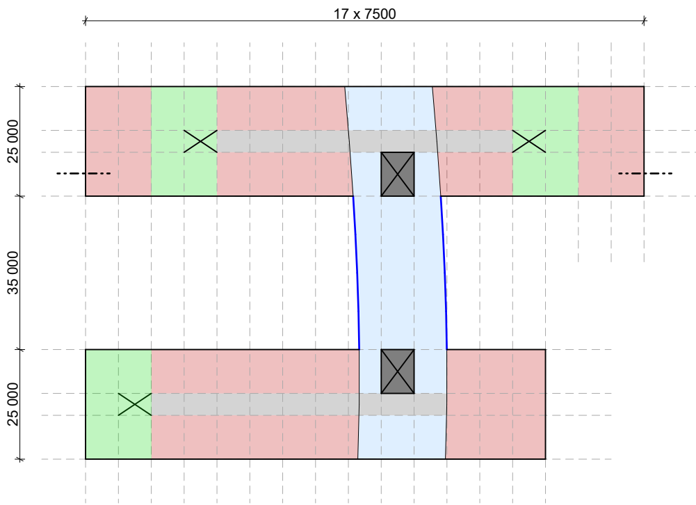
PÔDORYS 5 NP / STRECHA
